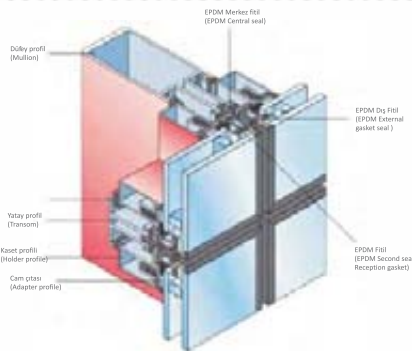
Silikon cephe , kompozit panel
